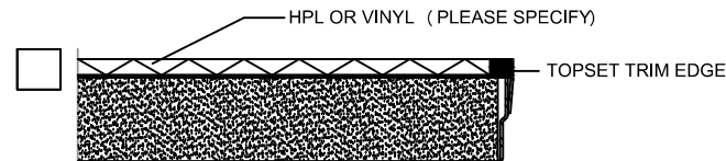
CORNER SECTION - TOPSET TRIM EDGE
